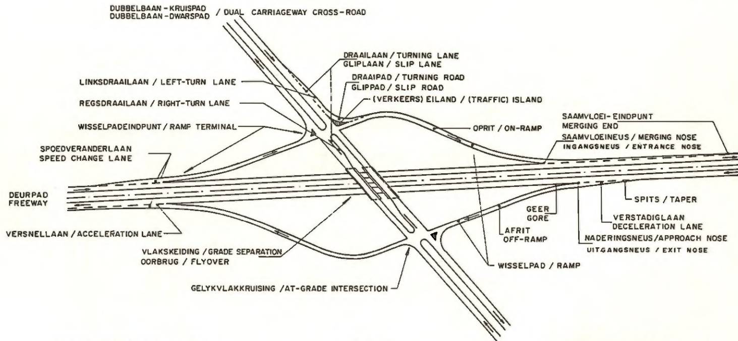
TOEGANGSWISSELAAR (DIAMANTTIPE)
