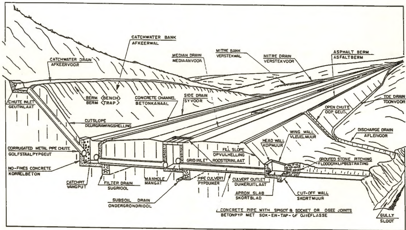
FIG. 4 ROAD DRAINAGE PADDREINERING (AUGUST/AUGUSTUS 1980)
