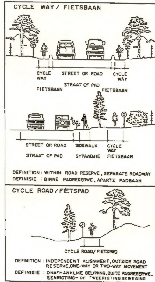
FIG. 6 CLASSIFICATION OF CYCLE PATHS KLASSIFIKASIE VAN FIETSPAAR
