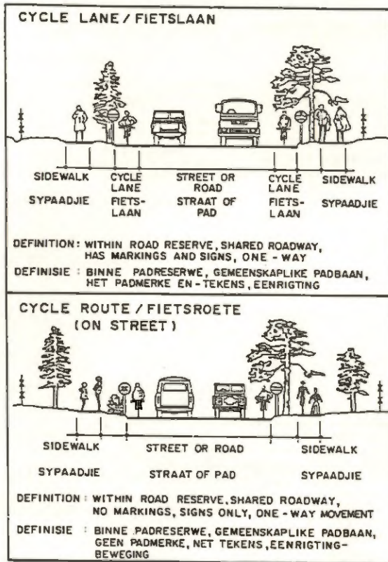
FIG. 6 CLASSIFICATION OF CYCLE PATHS KLASSIFIKASIE VAN FIETSPAAR
