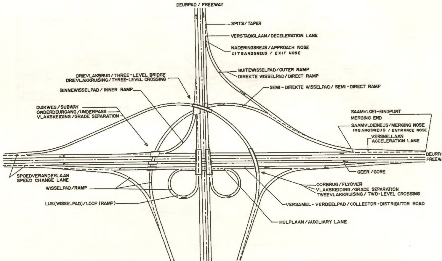
STELSELWISSELAAR (SEMI-DIREKTE TIPE MET TWEELUSSE)
